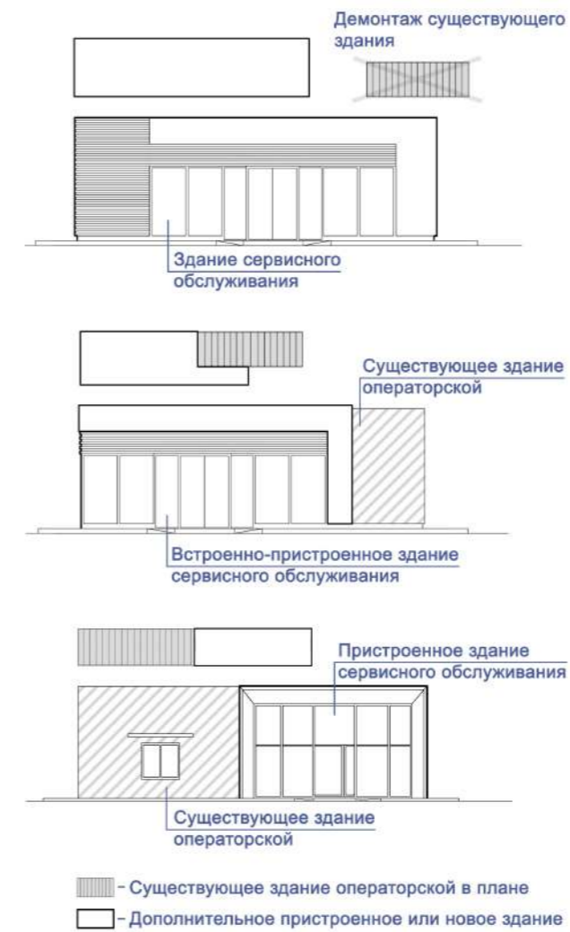
Вариант внешнего вида операторской АЗС в случае строительства нового здания.
