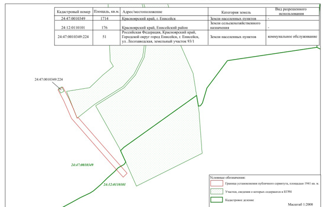
СХЕМА ГРАНИЦ ПУБЛИЧНОГО СЕРВИТУТА НА КАДАСТРОВЫЙ ПЛАН ТЕРРИТОРИИ «Строительство ЛЭП-10 кВ, КТП 10/0,4 кВ для электроснабжения объекта по адресу: г. Енисейск, ул. Лесозаводская 93/1»
